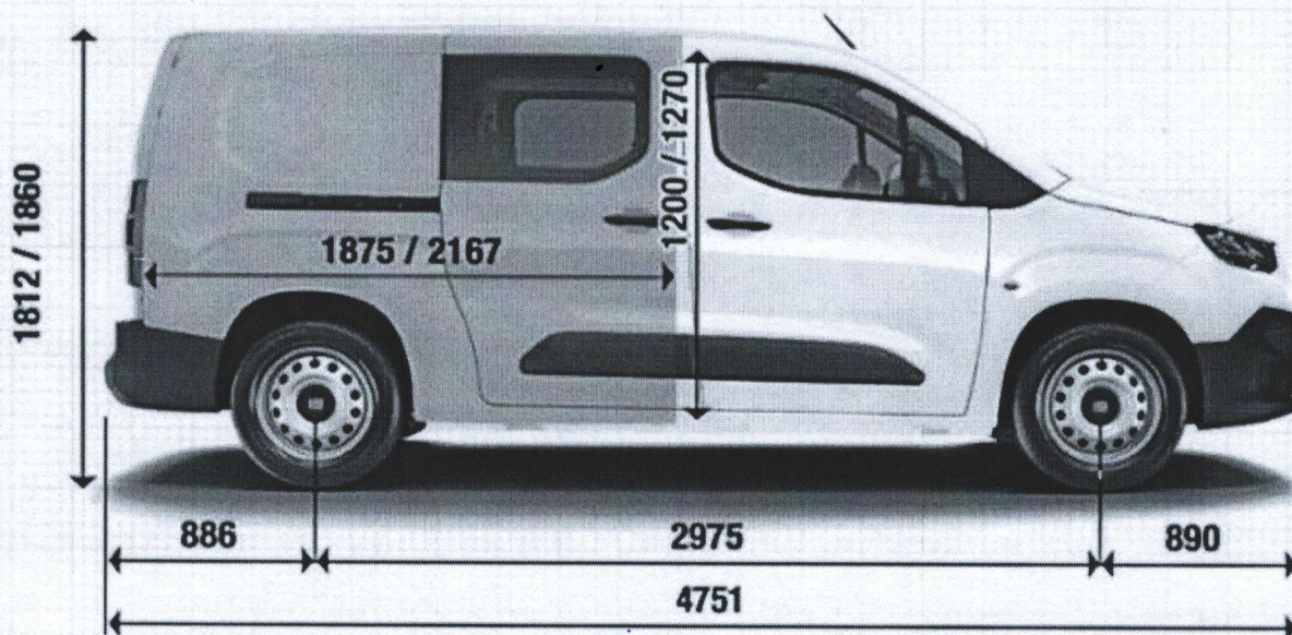
Габаритні розміри, мм
